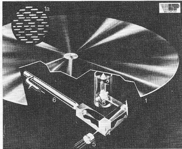
Afb. 2. Schematische opbouw van de VLP platenspeler: (1) VLP, (1a) kuiltjespatroon, (3) beweegbaar en kantelbaar spiegeltje, (4) halfdoorlatende spiegel, (5) foto-detector, (6) laser.
