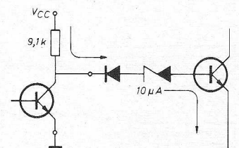
Fig. 5. „Passive pull-up” uitgang. De lekstroom, die de uitgang moet leveren aan 1 UL is hier aangegeven.
