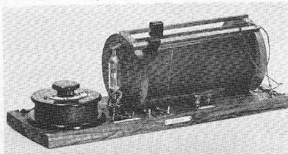
Afb. hieronder: Een door de firma Bal te Breda in 1919 vervaardigde ontvanger, met één „Bal” lampdetector, geannonceerd als: „Simplex” (Golflengten 600...8000 m). Een krachtig werkend amateurapparaat. Foto's: Universiteitsmuseum, Jac. P. Stolp.
