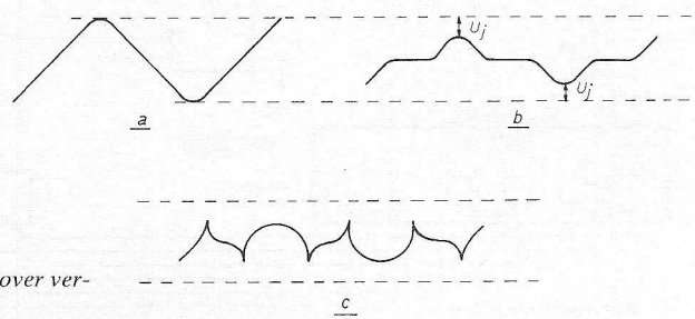
Fig. 9. Complementaire trap zonder nulstroominstelling.
