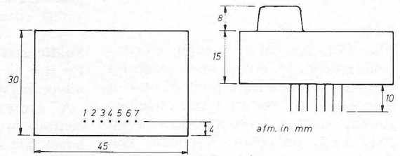
Fig. 1. Gasdetector als „black-box”.
