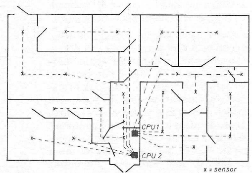
Fig. 5. Opstelling van sensoren in enkele ruimten.
