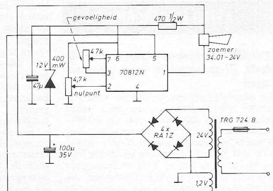
Fig. 3. Eenvoudige detector met gloei-wisselspanning en instelbare gevoeligheid.
