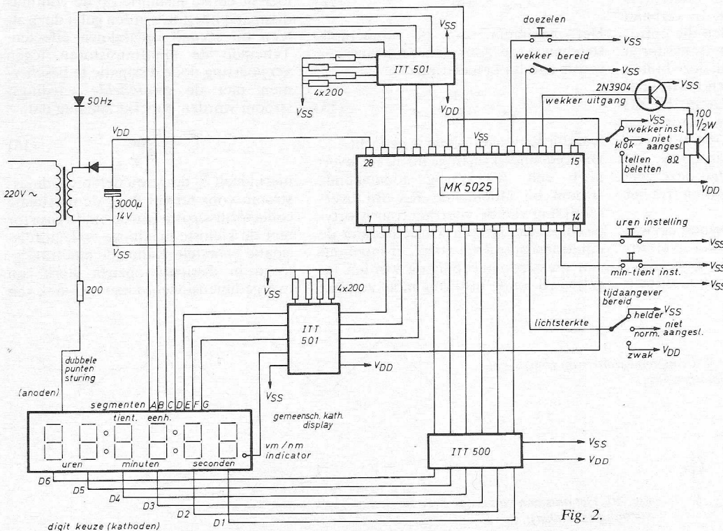
Fig. 1: Blokschema van de bouwsteen (boven). Fig. 2 geeft een voorbeeld van een complete schakeling om een klok met wek-mogelijkheid te realiseren.
