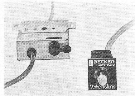
Afb. 6. De Verkehrsfunkadapter VA2 van Becker geeft een optische indicatie indien een verkeerszender wordt ontvangen. Bovendien is het mogelijk alleen die zenders hoorbaar te maken, die regelmatig verkeersberichten uitzenden.
