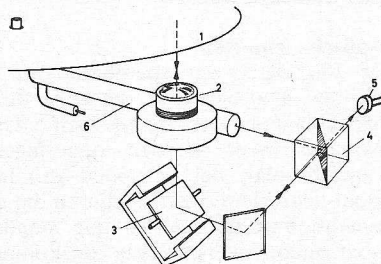
Fig. 5. Het optisch systeem, schematisch weergegeven: (1) VLP, (2) objectief, (3) kantelbaar spiegelje, (4) halfdoorlatende spiegel, (5) detector en (6) laser.
