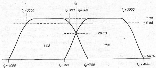
Fig. 3- Eisen, waaraan het filter moet voldoen.
