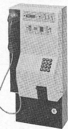
Munttelefoontoestel NT2000 voor Europees verkeer: de logische schakelingen zijn opgebouwd met MOS-componenten; zouden relais zijn toegepast dan zou het toestel een ruimte van 3 m 2 (ofwel een „celvol”) hebben ingenomen...
