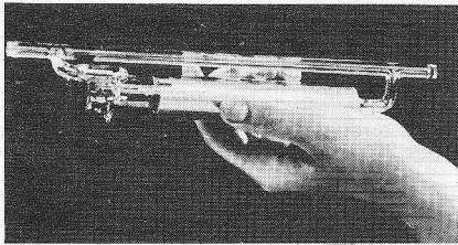
Afb. 4. De lichtbron van de VLP platenspeler is een He-Ne laser.
