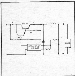
schakelende spanningsregulators
