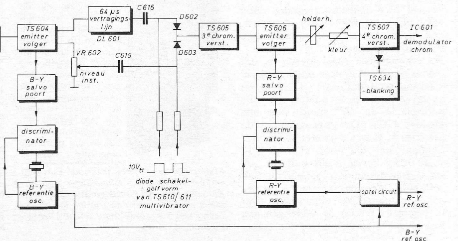
Fig. 1. Blokschema van de chrominantie- en dubbele referentie-oscillatorschakeling, zoals toegepast in de Mitsubishi CT-200B ontvanger. De vertragslijn en dioden D602/603 bewerkstelligen PAL/NTSC-omzetting en als het salvo vanaf TS605 op + of -45° van de normale -U positie staan, afhankelijk van de bistabiele fase, wordt het signaal van de referentie oscillator toegevoerd aan de (R-Y)-demodulator in IC601, in overeenkomstige fase verkregen door een deel van de (B-Y)-referentie oscillator toe te voeren aan die van de nominale (R-Y)-referentie oscillator.
