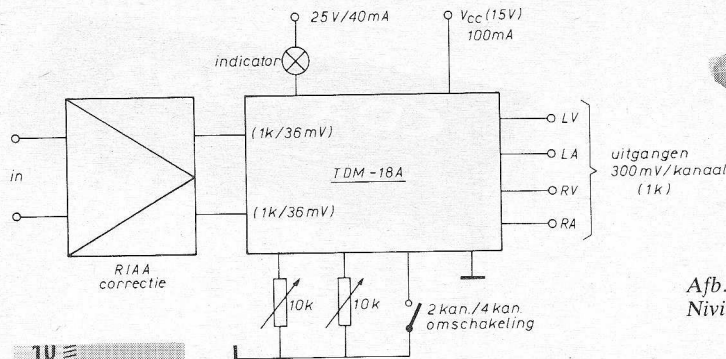
Fig. 2. Principe van de TMD-18A
