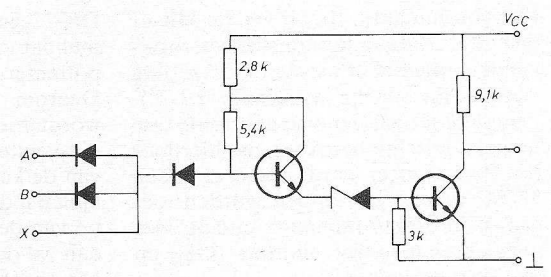
Fig. 7b is de configuratie voor een HiNIL passive pull-up NAND.
